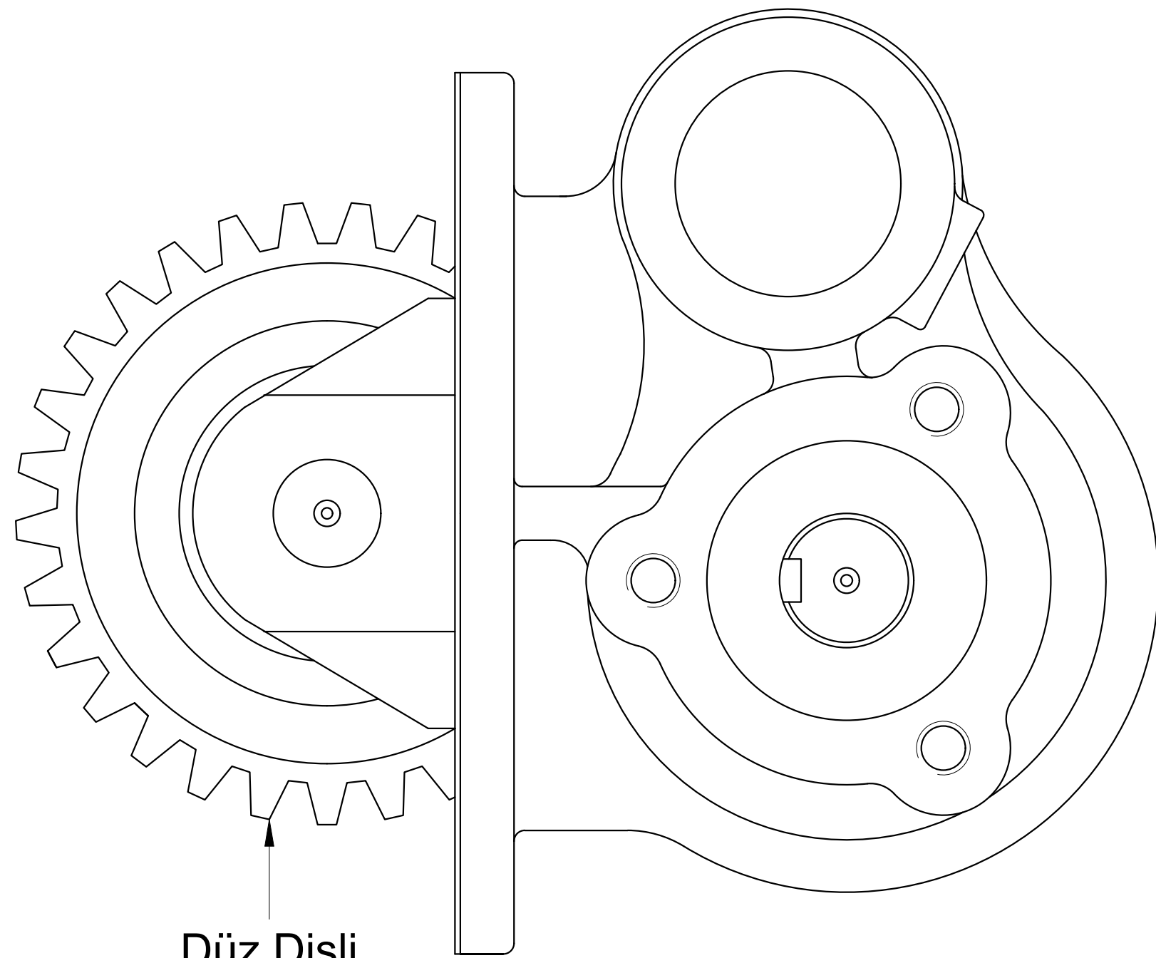
Düz Dişli Z=21
