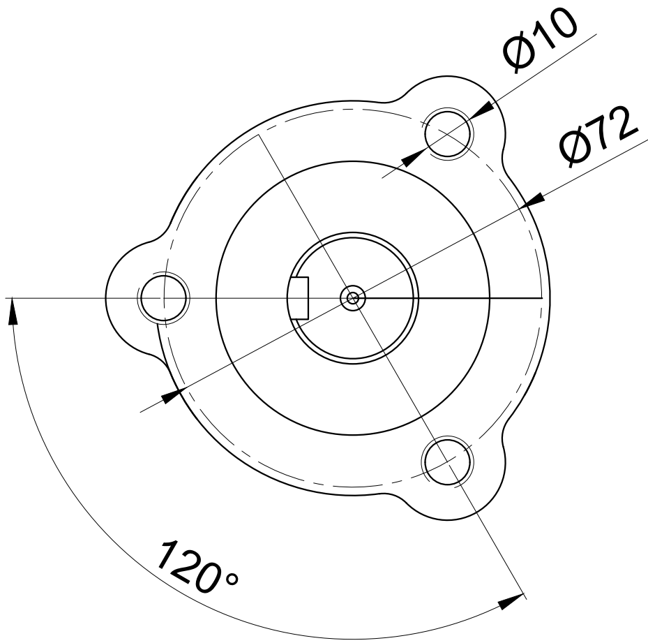
PTO Bağlantı Yeri Aracın Sağ ve Sol Yanı
